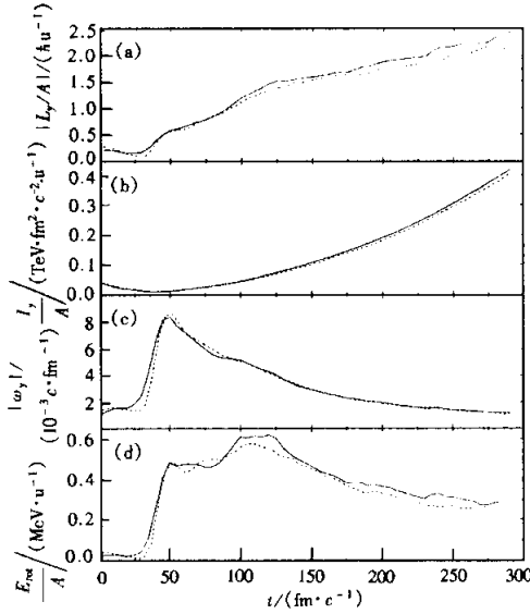
图 3 入射能量为 40\text{MeV/u} 及碰撞参数 b = 4\text{fm} 时 ^{58}\text{Fe} + ^{58}\text{Fe} (——) 和 ^{58}\text{Ni} + ^{58}\text{Ni} (.....) 的中间快度核子的 |L_y/A| , I_y/A , |\omega_y| 以及 E_{\text{rot}}/A 随时间的演化
