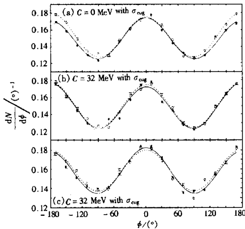
图 4 使用不同的对称能强度 C 和参数化的截面, 用 IQMD 模型预言的 ^{58}\text{Fe} + ^{58}\text{Fe} (●) 和 ^{58}\text{Ni} + ^{58}\text{Ni} (○) 在能量为 40\text{MeV/u} 碰撞参数 b = 4\text{fm} 时核子的方位角分布 (a) ^{58}\text{Fe} + ^{58}\text{Fe} : a_1 = 0.01081 , a_2 = 0.16003 ; ^{58}\text{Ni} + ^{58}\text{Ni} : a_1 = -0.01764 , a_2 = 0.16601 . (b) ^{58}\text{Fe} + ^{58}\text{Fe} : a_1 = -0.01506 , a_2 = 0.17152 ; ^{58}\text{Ni} + ^{58}\text{Ni} : a_1 = -0.01089 , a_2 = 0.17249 . (c) ^{58}\text{Fe} + ^{58}\text{Fe} : a_1 = 0.01143 , a_2 = 0.14593 ; ^{58}\text{Ni} + ^{58}\text{Ni} : a_1 = -0.00171 , a_2 = 0.13634 .
