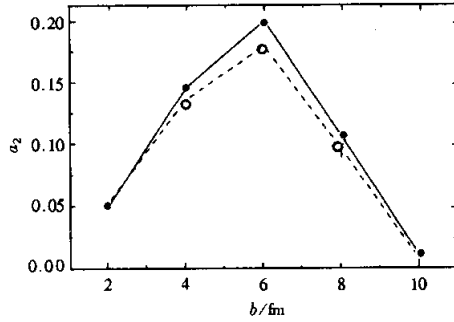
图 2 IQMD 模型预言的入射能量为 40MeV/u ^{58}\text{Fe} + ^{58}\text{Fe} (●)和 ^{58}\text{Ni} + ^{58}\text{Ni} (○)的中间速度的核子的 a_2 值随碰撞参数 b 的变化
