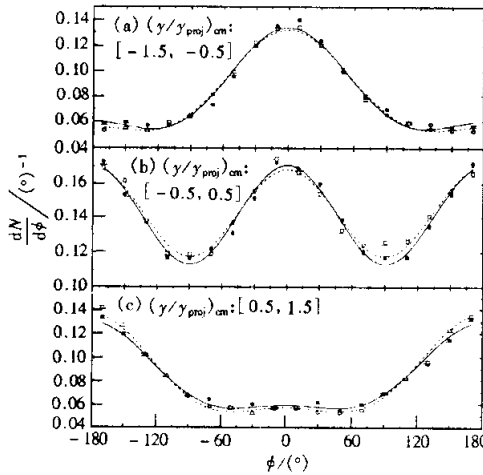
图 1 IQMD 模型预言的在 40MeV/u 的能量和碰撞参数 b = 6\text{fm} 下反应 ^{58}\text{Fe} + ^{58}\text{Fe} (●) 和 ^{58}\text{Ni} + ^{58}\text{Ni} (○) 的所有出射粒子的方位角分布 dN/d\Phi ——用(5)式拟合的 ^{58}\text{Fe} + ^{58}\text{Fe} 结果,.....用(5)式拟合的 ^{58}\text{Ni} + ^{58}\text{Ni} 结果.
