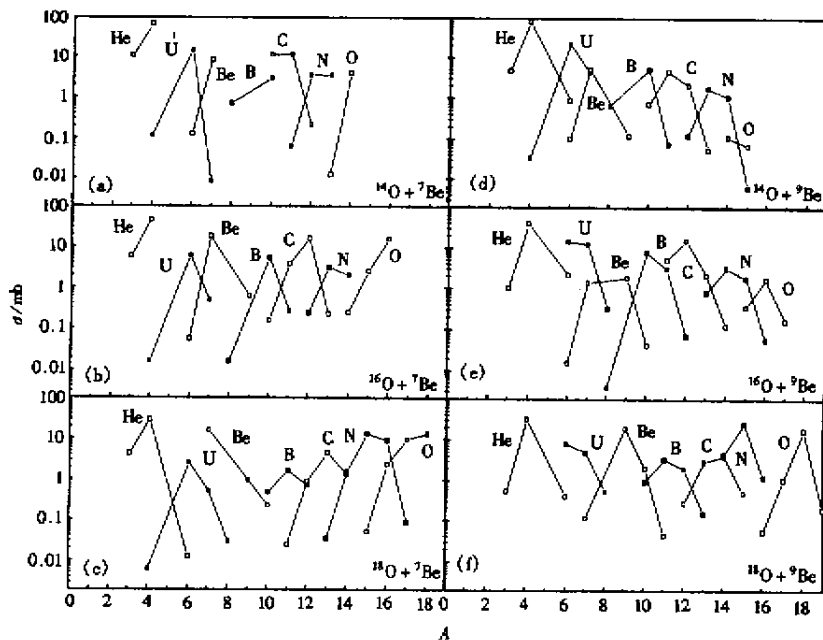
图 1 28.7MeV/u ^{14,16,18}\text{O} + ^7\text{Be} 生成核素的产生截面随同位素质量的变化关系
