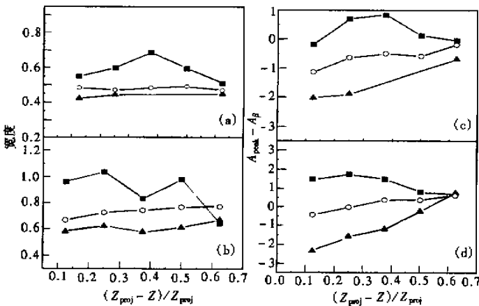
图 2 在 ^{14,16,18}\text{O} + ^7\text{Be} 反应中,所产生同位素分布的宽度(a)(b)和峰位与稳定同位素的质量差 \Delta A = A_{\text{peak}} - A_{\beta} (c)(d)随 (Z_{\text{proj}} - Z)/Z_{\text{proj}} 的变化关系
