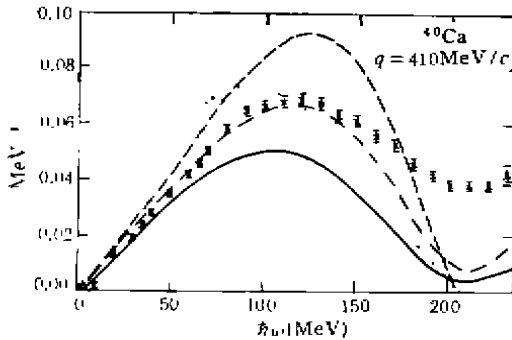
图1 q = 410\text{MeV}/c 时 ^{40}\text{Ca} 的横向响应函数 实验值取自文献[10]。点线: 壳模型; 虚线: 不含 \Delta 的 RPA, M^*(\varepsilon) ; 点-虚线: 含 \Delta 的 RPA, M^*(\varepsilon) ; 实 线: 含 \Delta 的 RPA, M^* = M 。
