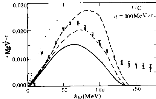
图2 q = 300\text{MeV}/c 时 ^{12}\text{C} 的横向响应函数 图例说明同图1
