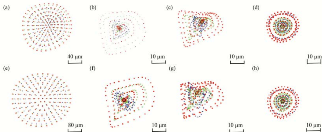
图4 -2D 和-5D 近视模型手术前后视网膜光斑分布 (a) -2D 模型手术前, (b) -2D 模型球面修正, (c) -2D 模型 Q 值优化修正, (d) -2D 模型波前像差引导修正, (e) -5D 模型手术前, (f) -5D 模型球面修正, (g) -5D 模型 Q 值优化修正, (h) -5D 模型波前像差引导修正
