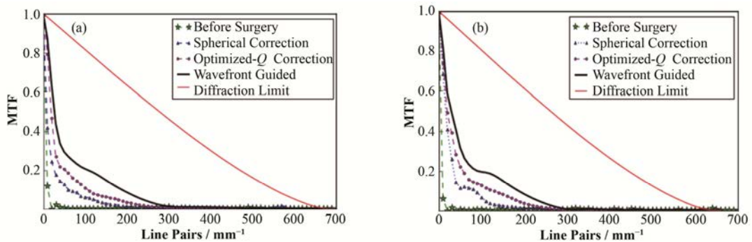
图 6 -2D (a)和-5D (b)模型手术前后 MTF 曲线的对比
