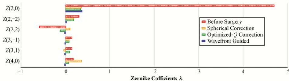
图7 -2D 模型(6 mm)不同手术前后各阶像差的变化
