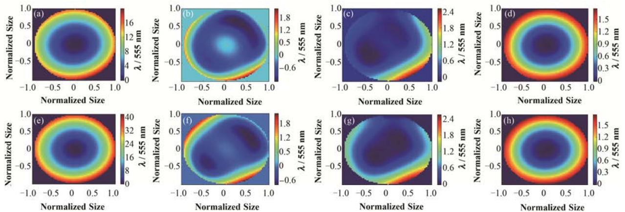
图 5 -2D 和-5D 模型手术前后波前像差的比较
