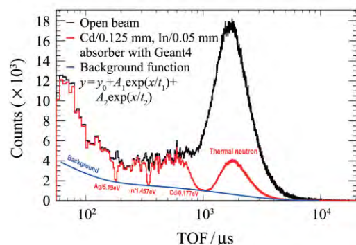
图 7 (在线彩图) Geant4 模拟的多吸收峰及本底函数拟合
