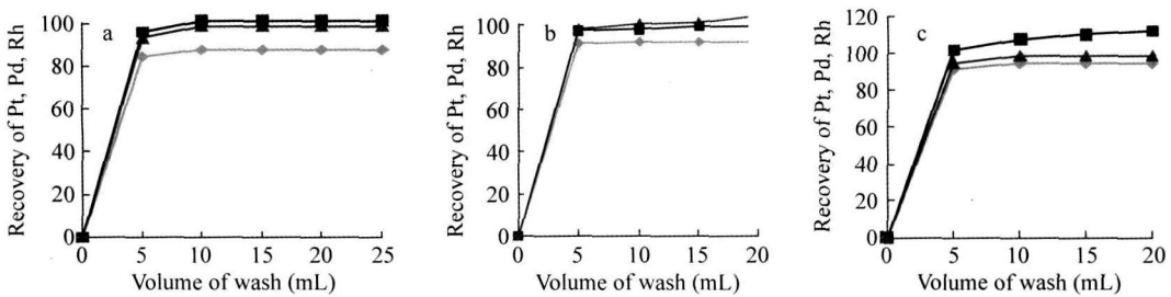
图 2 分离柱树脂高度 3 cm (a)、4 cm (b) 和 5 cm (c) 时铂族元素回收率
