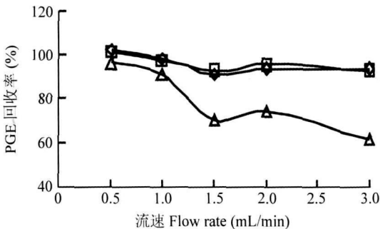
图 3 铂、钯、铑的回收率与流出液流速的关系
