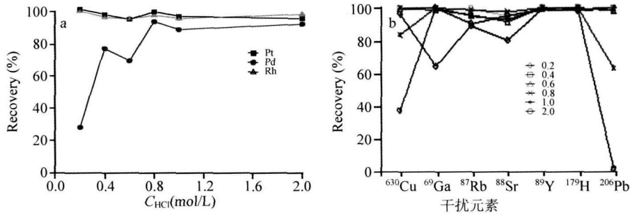
图 1 HCl 浓度对 Pt Pd Rh 回收率 (a) 和干扰元素分离效率 (b) 的影响
