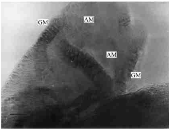
图1 超声波处理高序石墨产生的碳多层封闭结构的高分辨透射电子显微镜图 标尺为10nm
