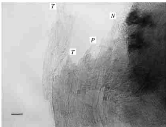
图2 在上述实验条件下形成的碳纳米管(T)、多面体(P)和巢式结构(N)等形成物的高分辨透射电子显微镜图 标尺为7nm
