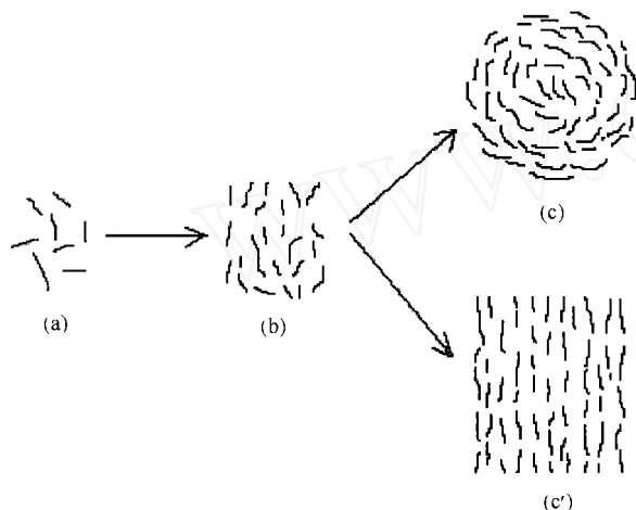
图 4 碳网络碎片在超声波处理水溶液中可能的聚集模式示意图 图 (a) 为各向同性排列, (b) 为二维向列, (c) 和 (c') 为三维向列
