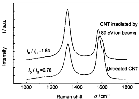
图3 初始碳纳米管和混合离子束 700 °C 处理 5 h 后样品的 Raman 光谱
