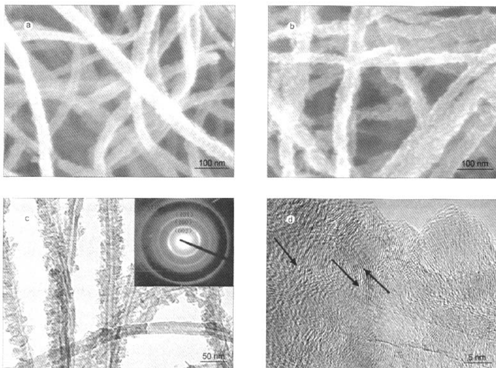
图2 80 eV混合离子700 °C处理后的CNTs表面形貌和微观结构。(a)处理1.5 h SEM图,处理5 h;(b)SEM图,(c)TEM图(内嵌为选区电子衍射图),(d)HRTEM图
