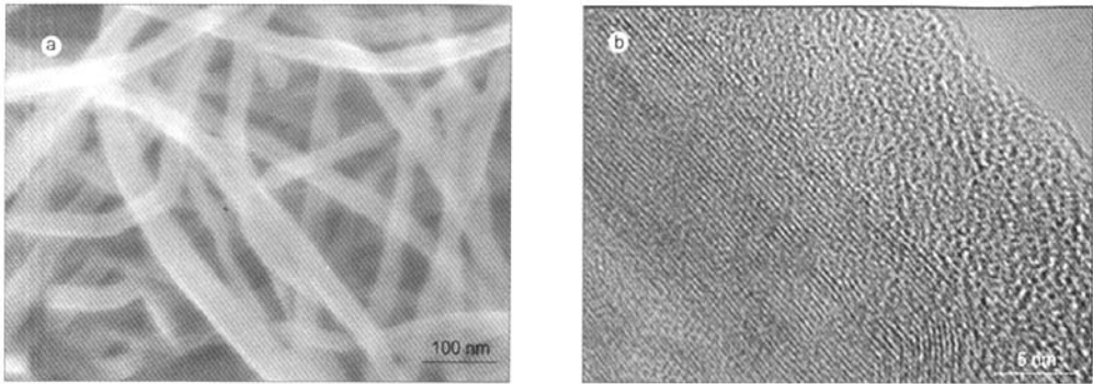
图4 300 °C处理 1.5 h 后的碳纳米管. (a) 典型的 SEM 图; (b) 典型的 HRTEM 图 Fig.4 CNTs treated at 300 °C for 1.5 h. (a) typical SEM image; (b) typical HRTEM image
