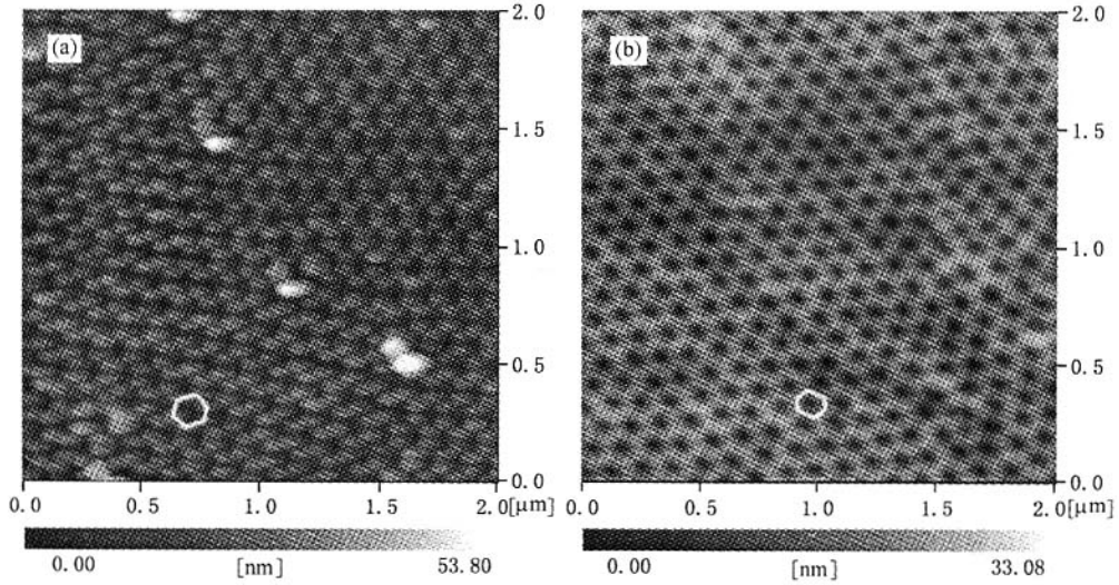
图 2 (a)溅射前 AAO 正面的 AFM 照片 (b)经 Ar^+ 束倾角 30^\circ 溅射(样品台旋转)后的 AAO 正面 AFM 照片
