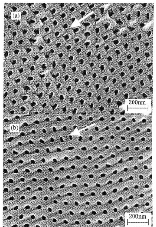
图 4 经 Ar^+ 束倾角溅射(样品台固定)后的 AAO 表面 SEM 照片 (a)倾角 45^\circ (b)倾角 60^\circ
