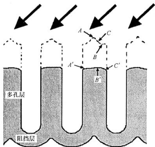
图5 \text{Ar}^+ 束倾角溅射 AAO 示意图
