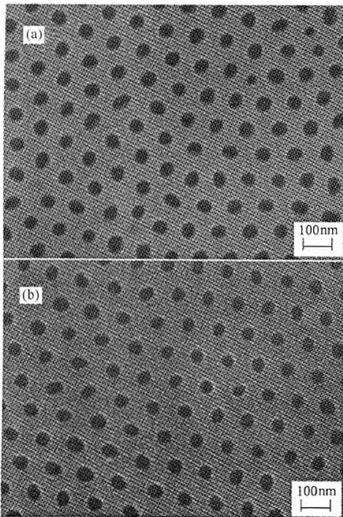
图 3 分别经 Ar^+ 束以 30^\circ 倾角刻蚀(样品台旋转)后的 AAO 正面(a)和反面(b)SEM 照片
