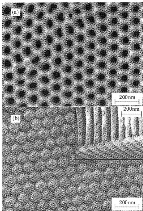
图 1 AAO 样品的 SEM 照片 (a)正面 (b)反面(阻挡层),插图 为侧面斜视图
