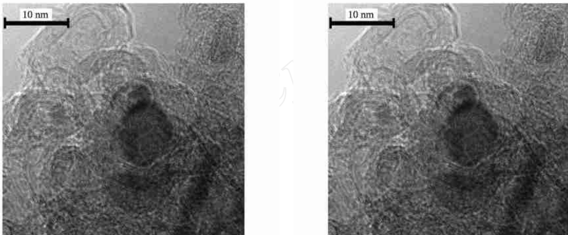
图 1 双离子( ^{40}\text{Ar}^+ , \text{C}_2\text{H}_6^+ )辐照 MWCNT 生成的金刚石纳米晶、碳洋葱和富勒烯三种结构典型的 TEM 照片
