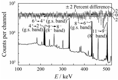
图 4 Ahmad 等 [47] 实验得到的能量在 100—500 keV 之间的 \gamma 射线谱
