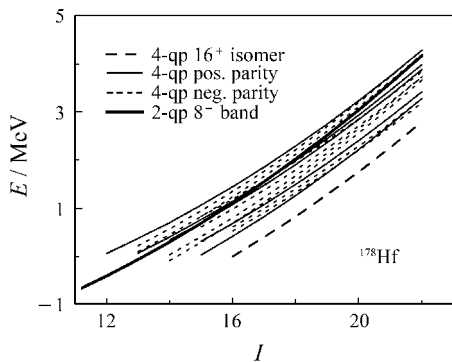
图 6 文献 [38] 中计算得到的 178 Hf m2 的同质异能态 16^+ 及其邻近的转动带能级
