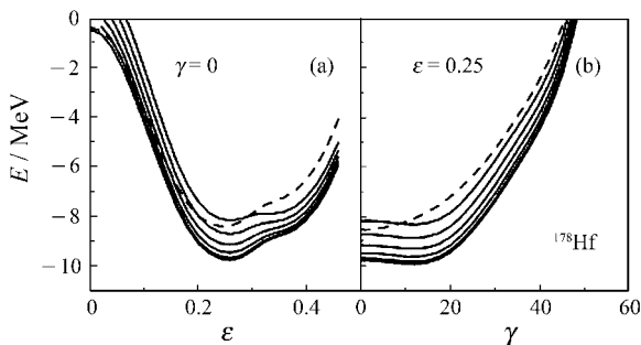
图 7 文献 [38] 中 178 Hf 的基态转动带的能量曲面 (a) 四极形变 \epsilon_2 , \gamma = 0 ; (b) \gamma 形变, \epsilon_2 = 0.25 ; -(\cdots) 对应于投影(未投影)的计算。
