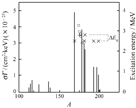
图 1 质子壳层 ( P < 82 ) 原子核的 ( \gamma, \gamma' ) 反应积分截面 (左轴) 与可能的 K 混合态的激发能 (右轴) [43]
