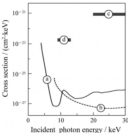
图 5 Ahmad 等 [45, 47, 48] 实验得到的截面与 Collins 等 [44, 46] 实验得到的截面的比较 入射的 X 射线光子的能量从 4 keV 到 30 keV。
