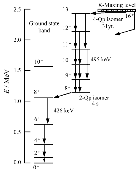
图 2 Collins 实验得到的 ^{178}\text{Hf} 的能级图 [44]
